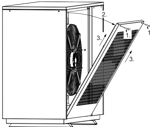
Rys. 7.1: Otwieranie kratownic
