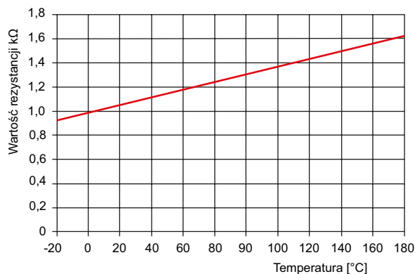
Rys. 7.10: Charakterystyka czujnika PT 1000
