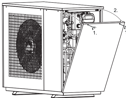
Rys. 7.2: Otwieranie bocznych osłon blaszanych, krok 1 i 2
