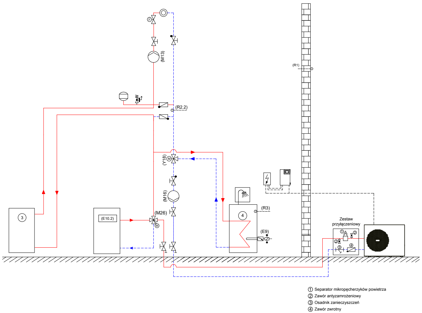
schemat hydrauliczny 2
