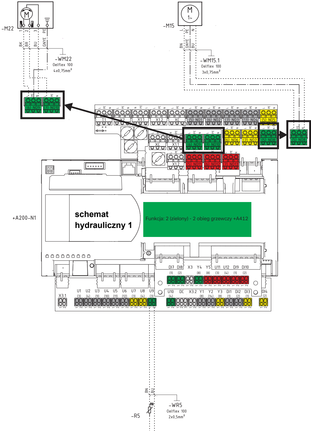
Czujnik 2 obiegu grzewczego
