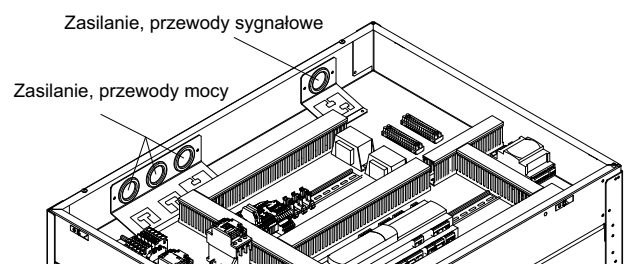
Rys. 7.3: Wpust kablowy do rozdzielni
