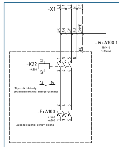
Rozdzielnia elektryczna
